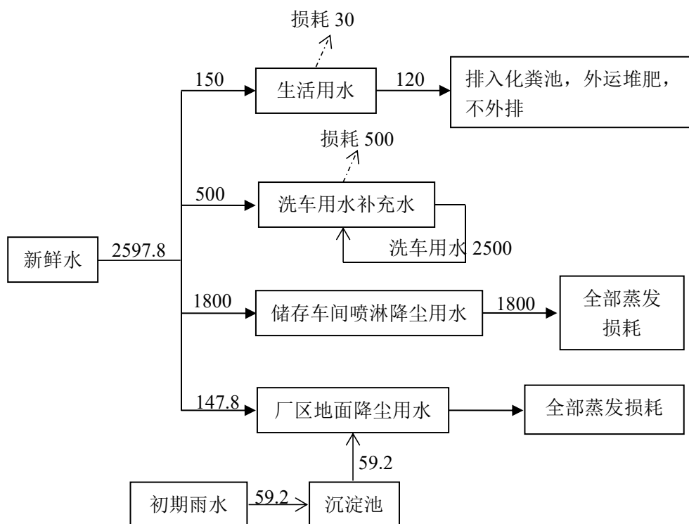
图 2-1 项目用水平衡图 单位：m 3 /a
