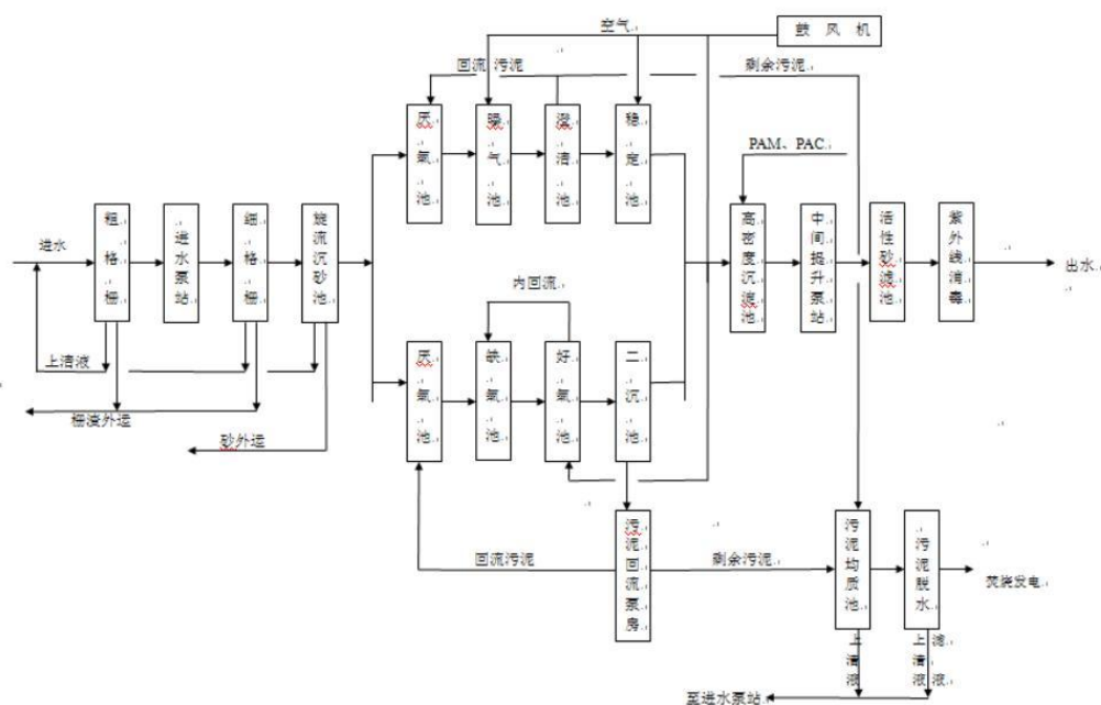
图 4-1 大禹污水处理厂工艺流程图
