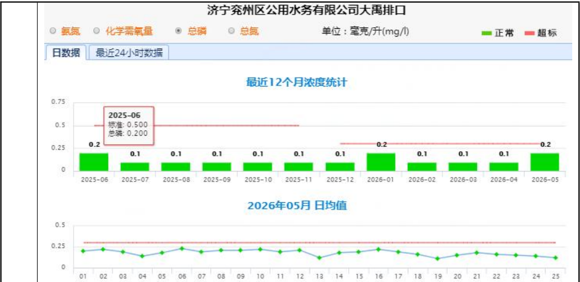
图 4-4 兖州大禹污水处理有限公司总磷排放情况（总磷 \leq 0.3\text{mg/L} ）
