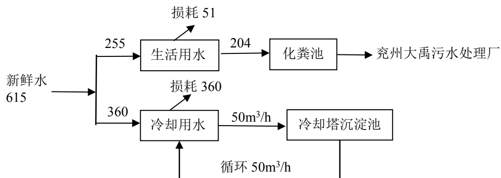
图 2-1 项目水平衡图 单位 m³/a
